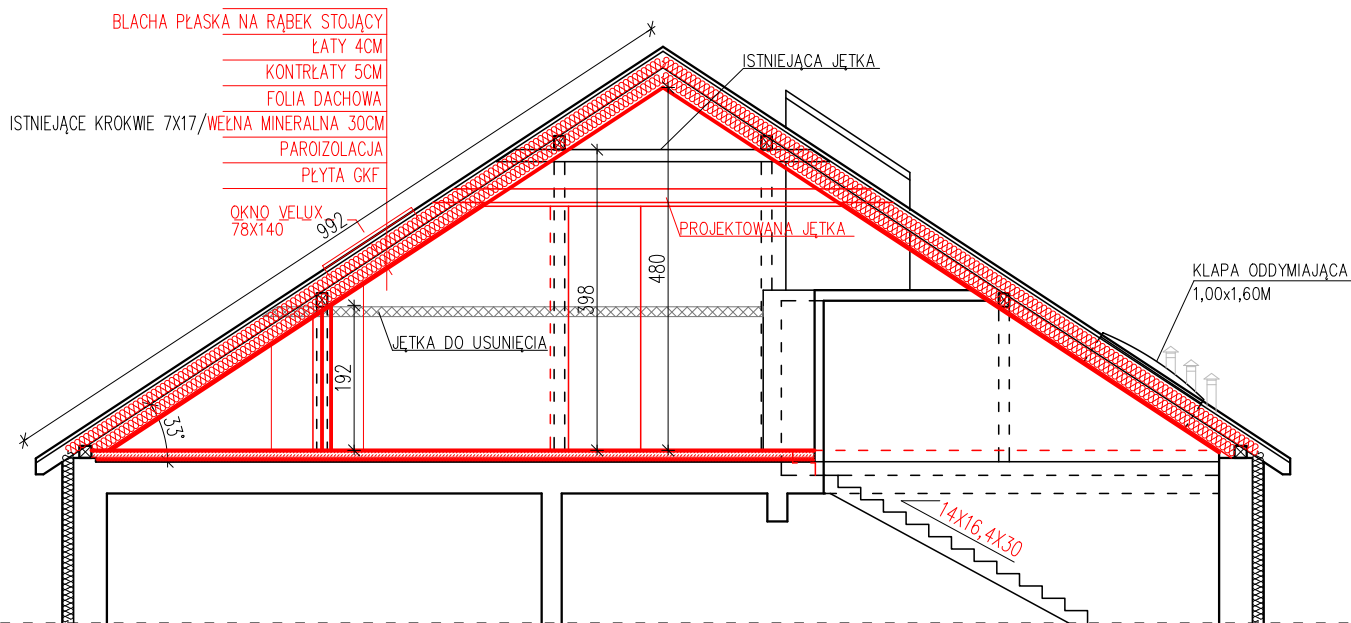
PRZEKRÓJ B-B
